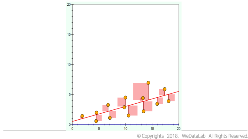
[그림 13] 잔차제곱합의 시각화 — Cost(\beta) = \sum (\hat{y}_i - y_i)^2 .
