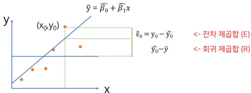
[그림 22] 잔차제곱합(E)과 회귀제곱합(R)의 시각화 .
