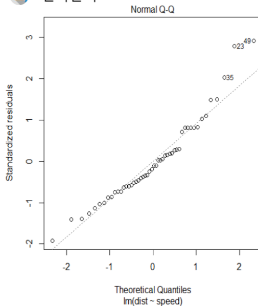
[그림 39] cars 데이터 잔차의 Q-Q plot — 양 끝 점들이 직선에서 살짝 벗어나지만 대부분은 직선 위에 있다.
