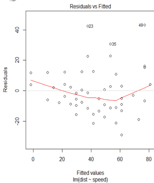
[그림 37] cars 데이터의 잔차도 — 적합값이 커질수록 잔차가 넓게 퍼진다(등분산성 의심).
