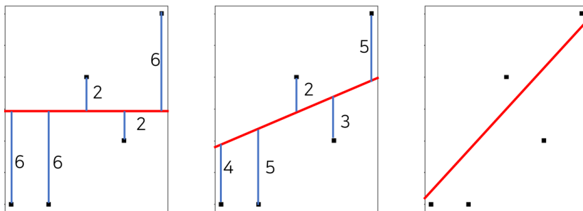
[그림 10] 후보 직선 2 — 잔차제곱합 = 4^2 + 5^2 + 2^2 + 3^2 + 5^2 = 79 .
